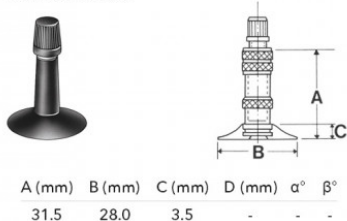
AV Schrader
